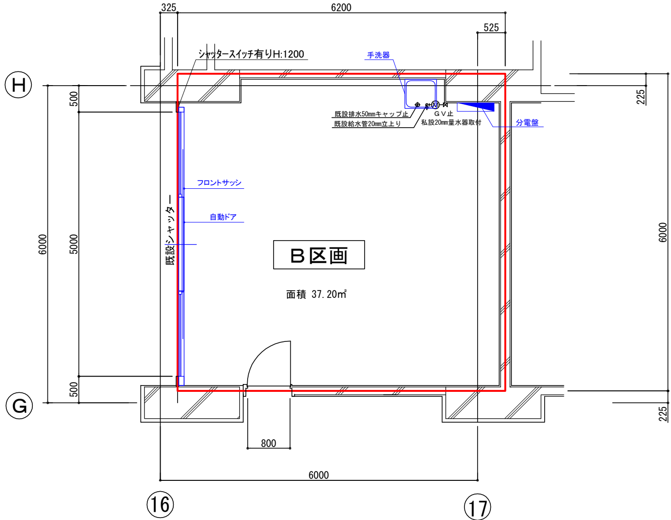
平面図 1/50
